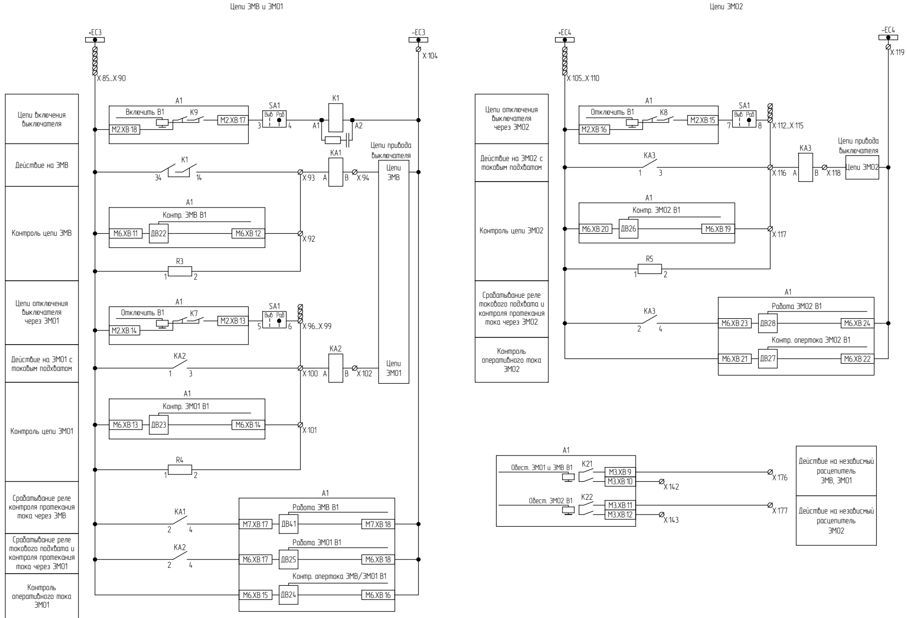
Рисунок В.3 – Схема электрическая принципиальная (часть 3)
