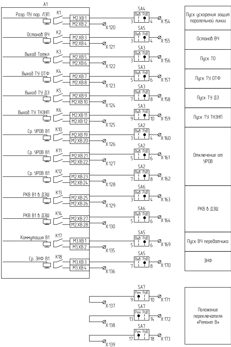
Рисунок В.4 – Схема электрическая принципиальная (часть 4)
