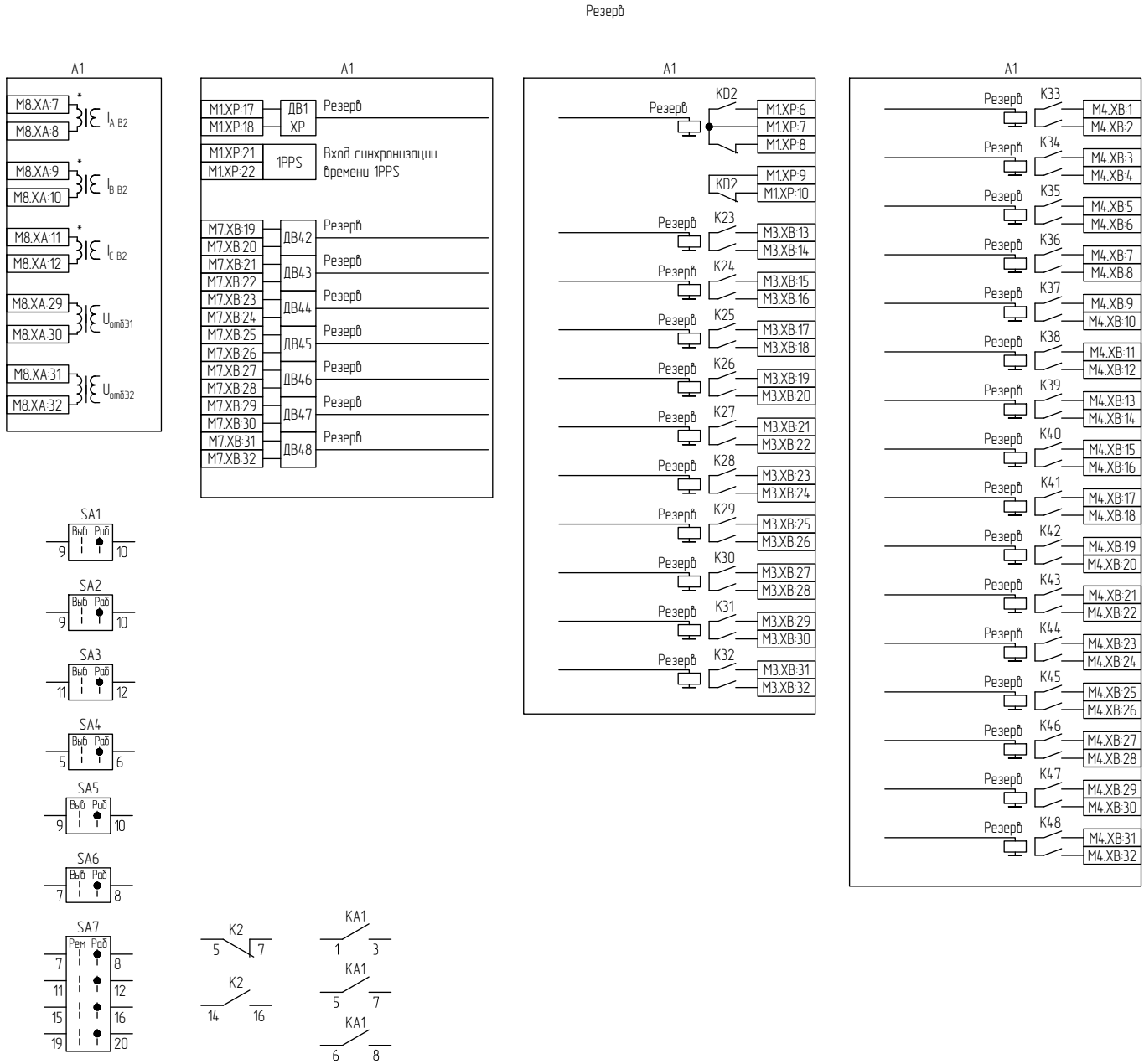
Рисунок В.6 – Схема электрическая принципиальная (часть 6)
